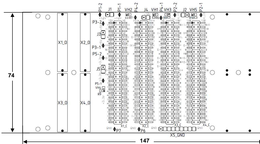
Расположение элементов на плате удлинителя
